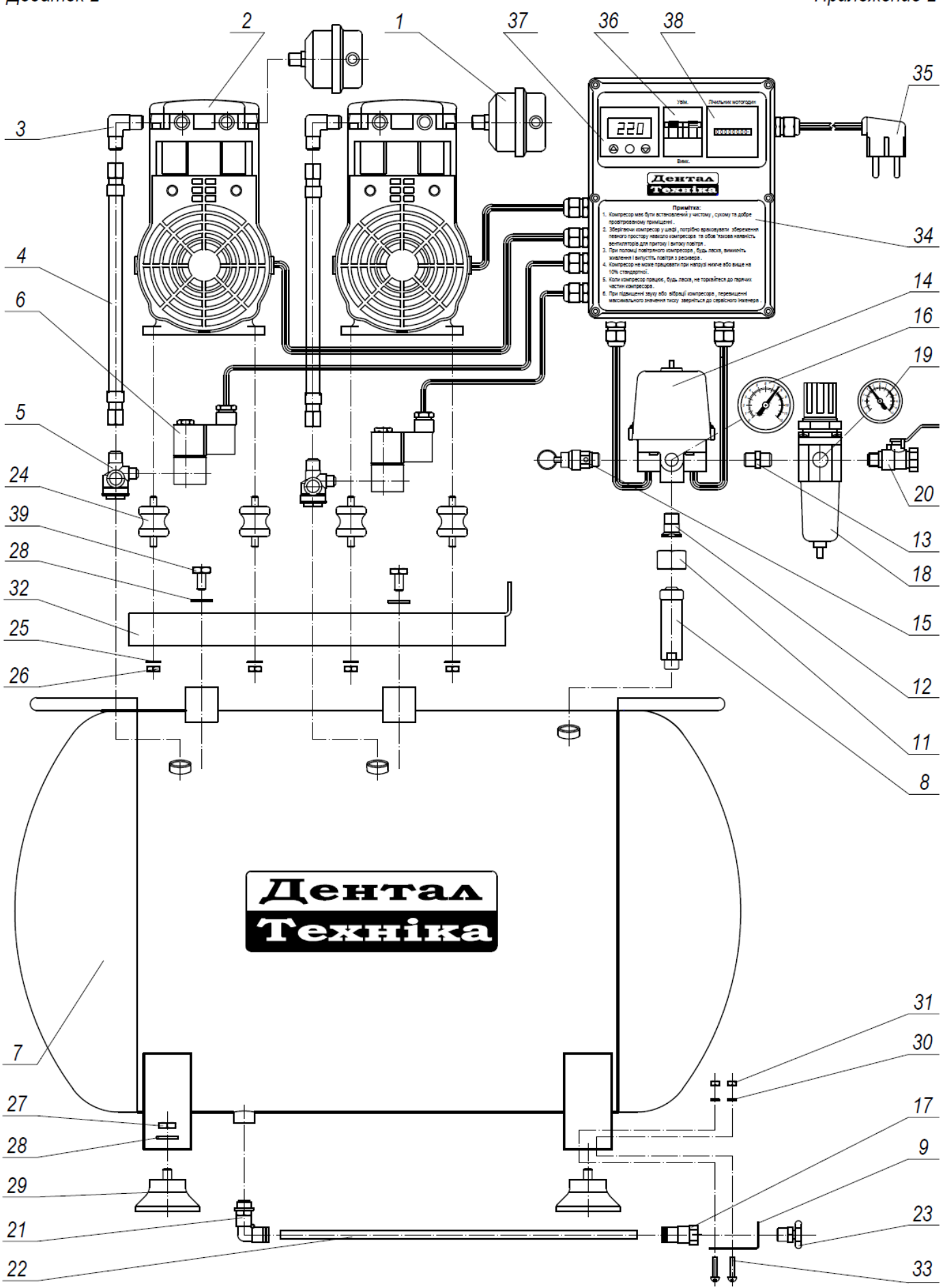
Малюнок 2: Схема з'єднань компресора ДТ750/2-65
