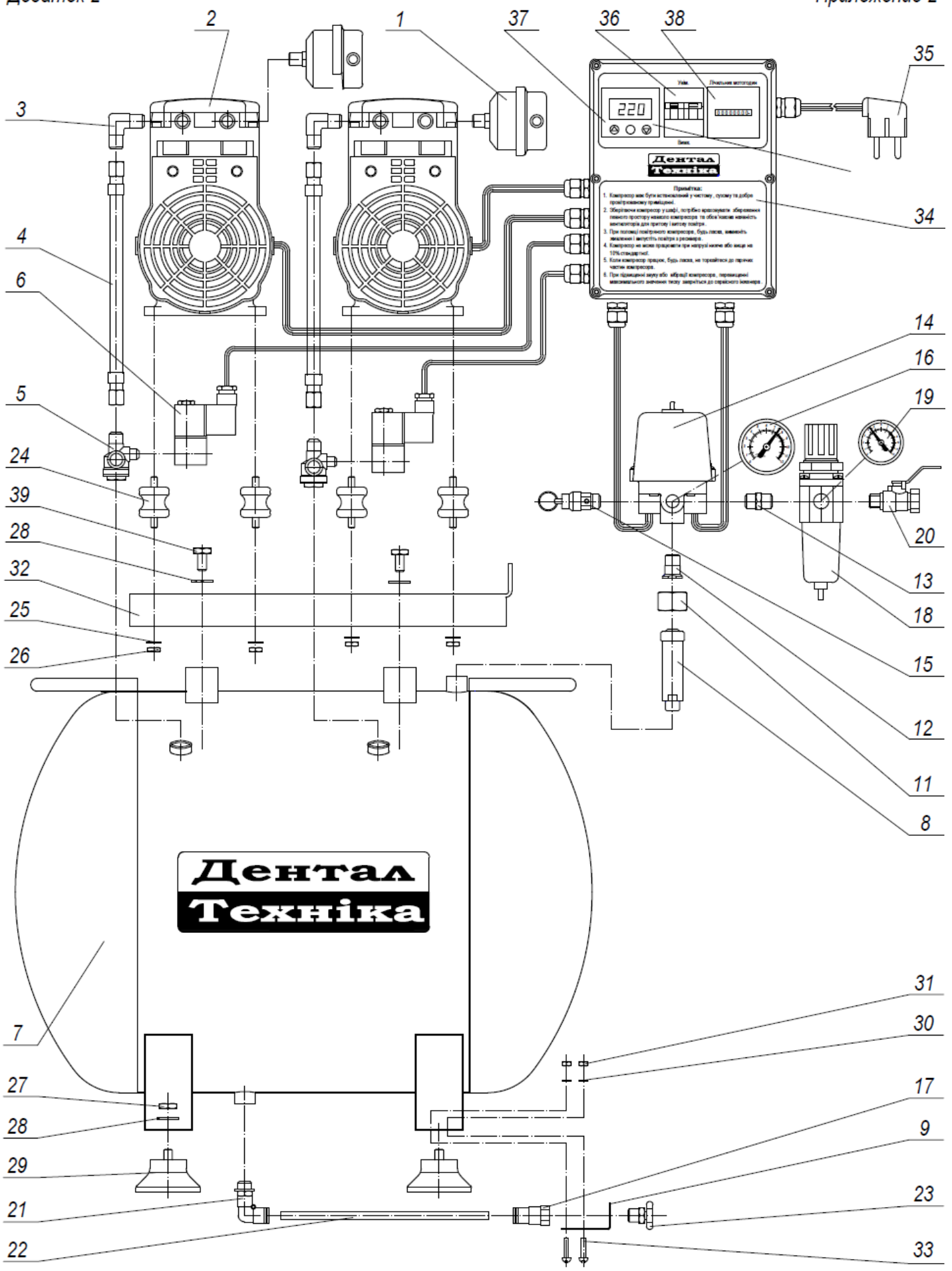
Малюнок 2: Схема з'єднань компресора ДТ550/2-50
