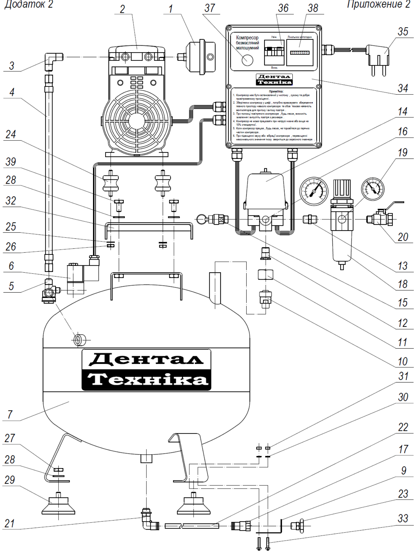
Малюнок 2: Схема з'єднань компрессора ДТ550/1-24
