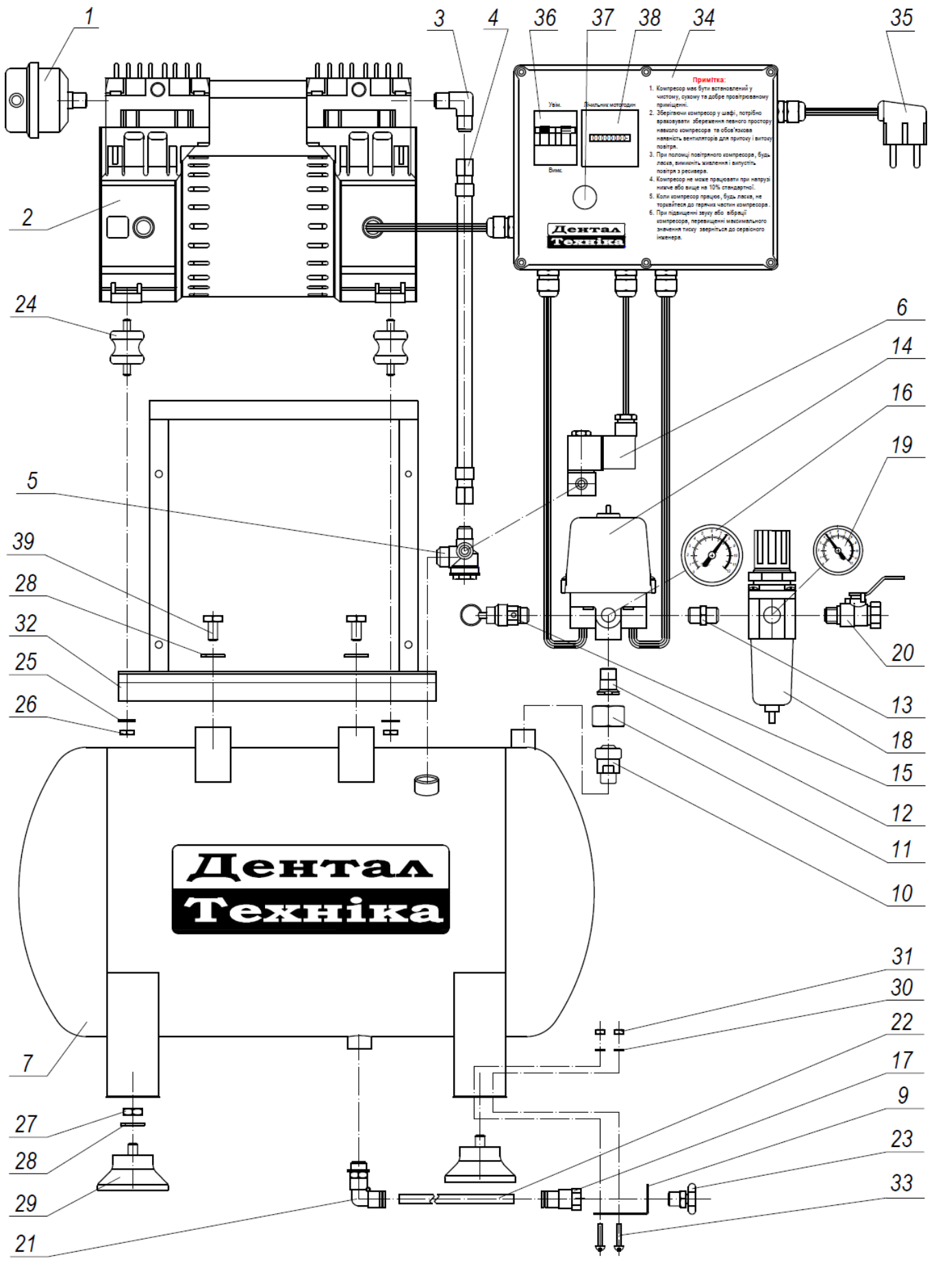
Малюнок 2: Схема з'єднань компресора ДТ550/1-24
