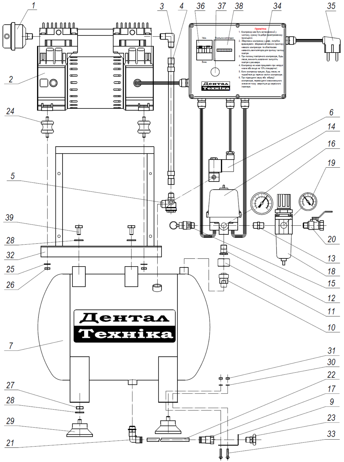
Малюнок 2: Схема з'єднань компресора ДТ550/1-16
