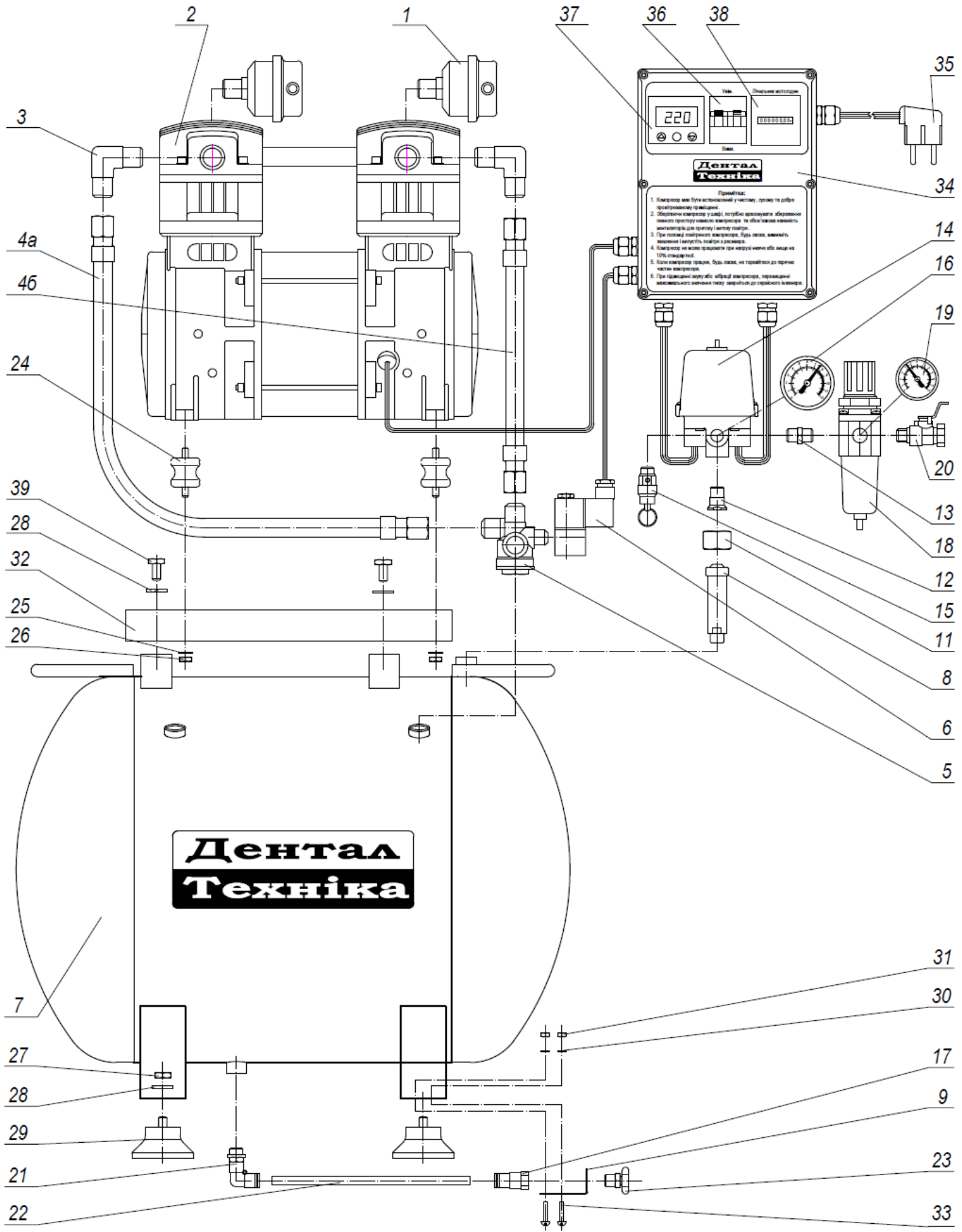
Малюнок 2: Схема з'єднань компресора ДТ1100/1-50
